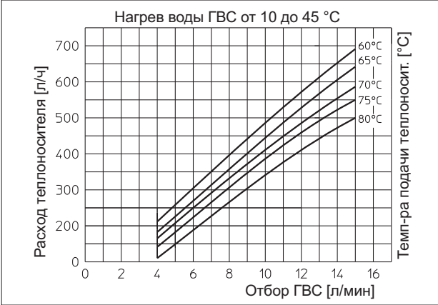
Расход теплоносителя – Класс мощности 2 – 15 л/мин
