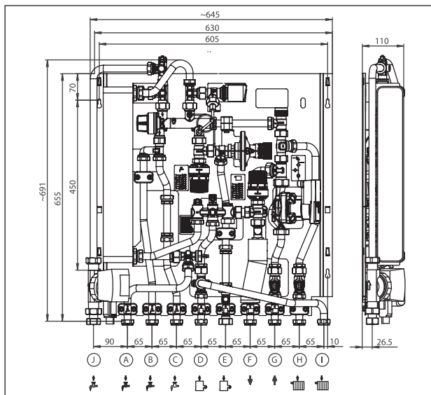
Размеры станции с прямым, смесительным отопительным контуром и циркуляцией
