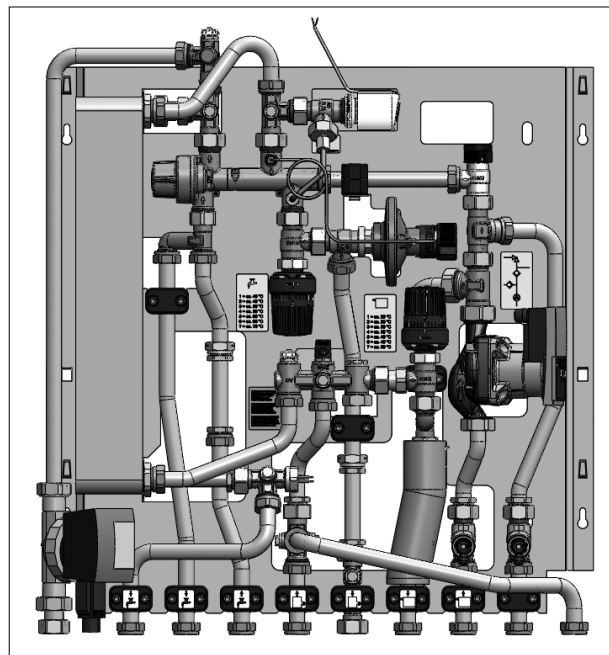
„Regudis W-HTF“ со смесительным, прямым отопительным контуром и циркуляционным трубопроводом
