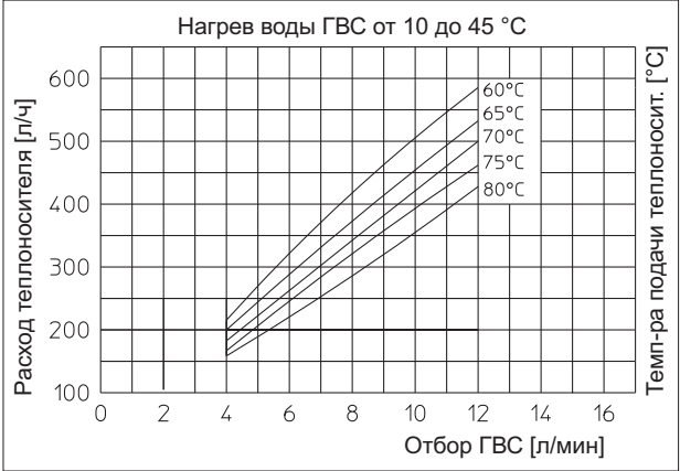
Расход теплоносителя – Класс мощности 1 – 12 л/мин
